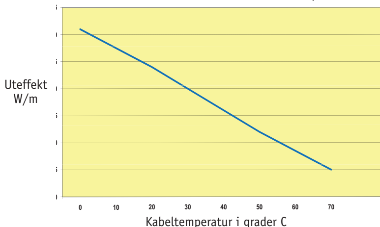
Nominell uteffekt för K4 vid olika kabeltemperaturer
